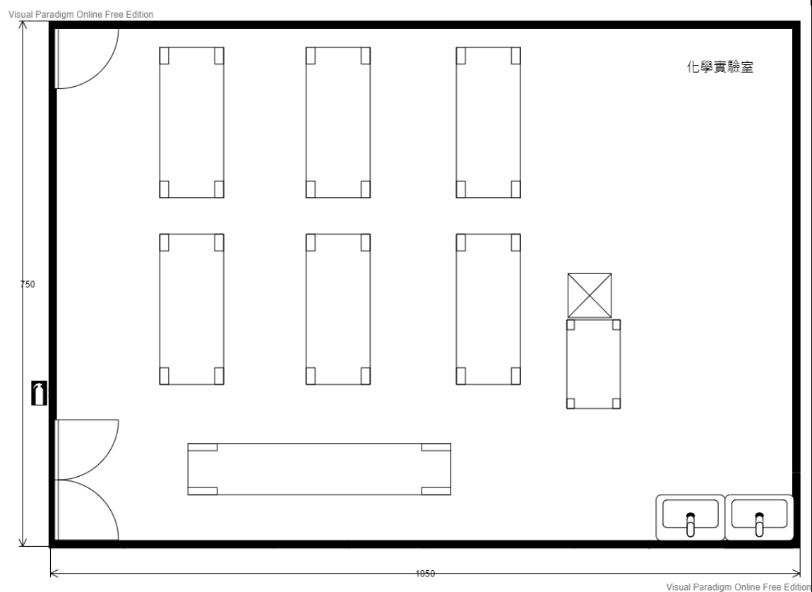
平面圖
